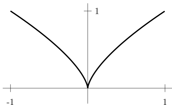
Abbildung 1: Die Kurve \gamma: [-1, 1] \rightarrow \mathbb{R}^2 , t \mapsto (t^3, t^2) , ist stetig differenzierbar, aber nicht glatt. Die Kurve \gamma^*: [-1, 1] \rightarrow \mathbb{R}^2 , t \mapsto (\text{sign}(t)|t|^{3/2}, |t|) ist eine stückweise glatte Umparametrisierung von \gamma .
