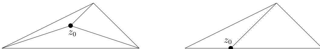
Abbildung 5: Unterteilung eines Dreiecks, welches z_0 enthält, in kleinere Dreiecke, welche z_0 als Eckpunkt haben.
