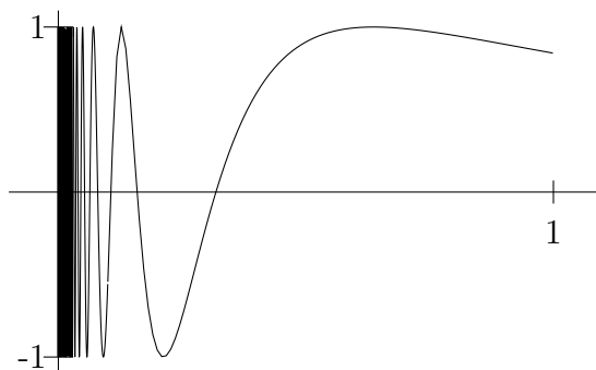
Abbildung 2: Die Menge \{(x, \sin(1/x)): 0 < x \leq 1\} \cup \{(0, y): -1 \leq y \leq 1\} ist zusammenhängend, aber nicht wegzusammenhängend.
