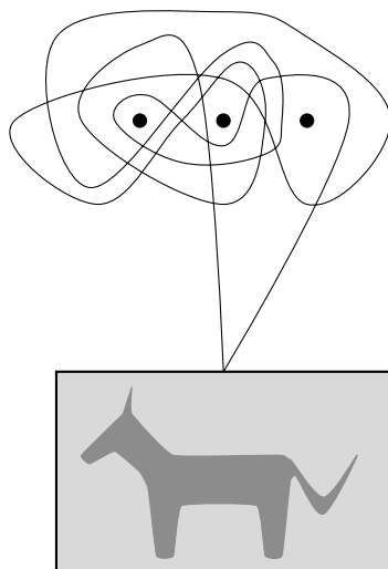
Abbildung 11: Ein an drei Nägeln aufgehängtes Bild.
