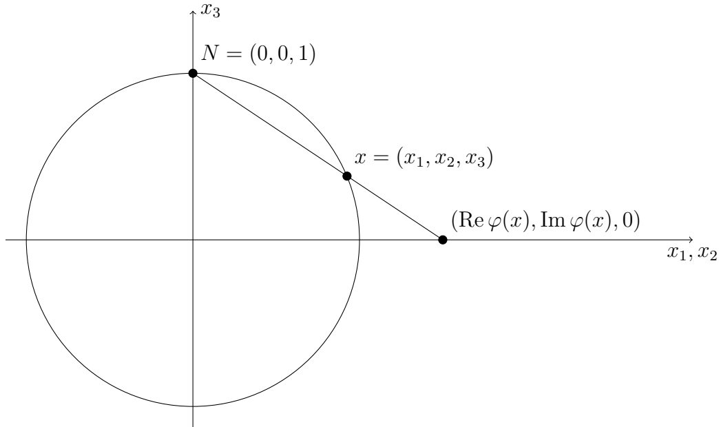
Abbildung 19: Die stereographische Projektion.
