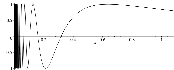
Abbildung 26: Eine zusammenhängende Menge.
