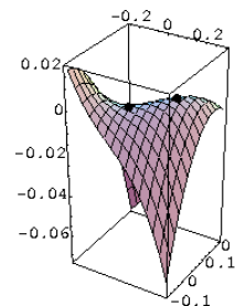
Abbildung 29: Der Graph der Funktion aus Beispiel 1.
