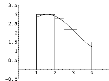
Abbildung 20: Eine Riemannsche Summe.
