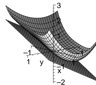
Abbildung 27: Approximation des Graphen durch eine Ebene.
