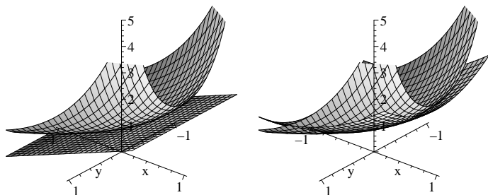
Abbildung 32: Taylorpolynome vom Grad 1 (links) und 2 (rechts).
