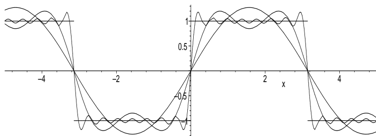
Abbildung 23: Fourierpolynome vom Grad 1, 3 und 15.
