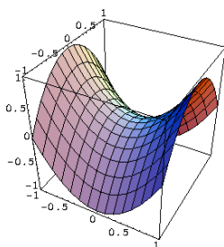
Abbildung 28: Ein Sattelpunkt.
