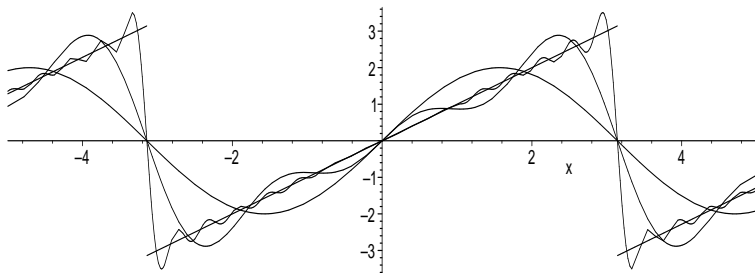
Abbildung 21: Fourierpolynome vom Grad 1, 3 und 15 für f(x) = x
