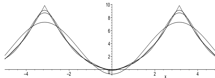
Abbildung 22: Fourierpolynome vom Grad 1, 3 und 5 für f(x) = x^2
