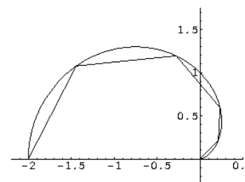
Abbildung 24: Approximation einer Kurve durch einen Streckenzug.
