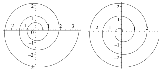
Abbildung 25: Logarithmische Spirale (links) und Archimedische Spirale (rechts).
