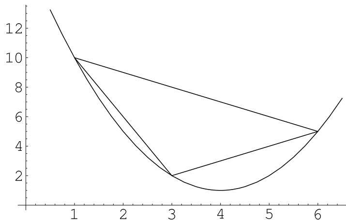
Abbildung 15: Konvexität.
